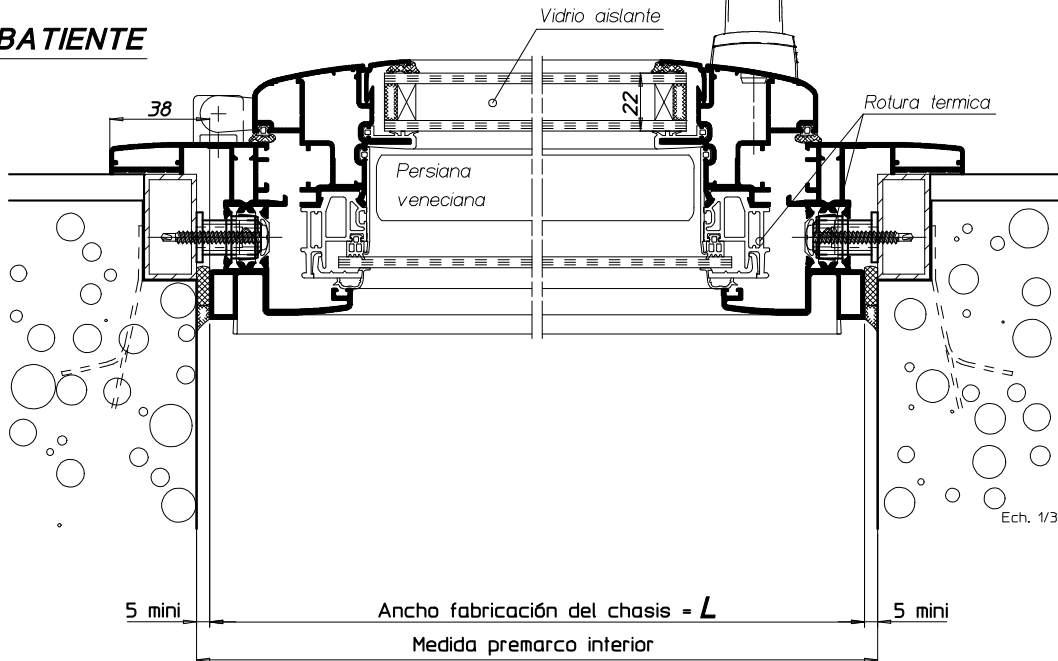
SECCIÓN HORIZONTAL
