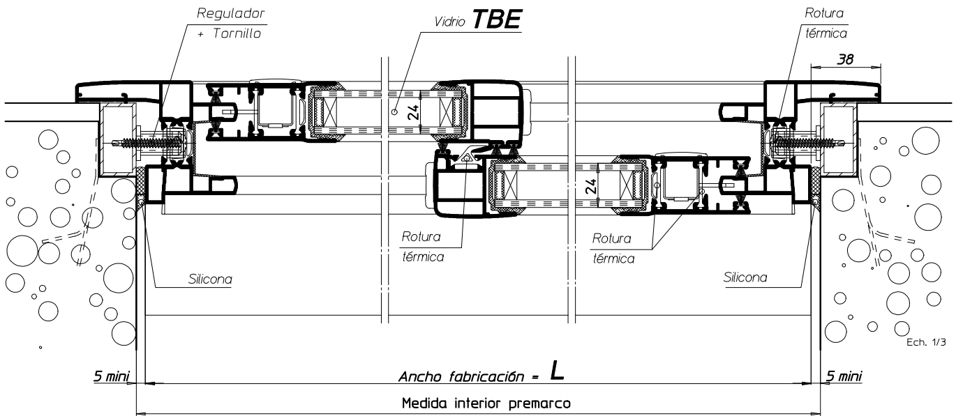
SECCIÓN HORIZONTAL
