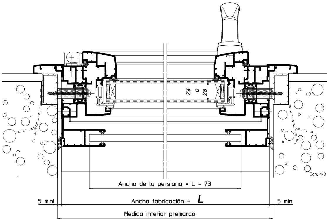
SECCIÓN HORIZONTAL
