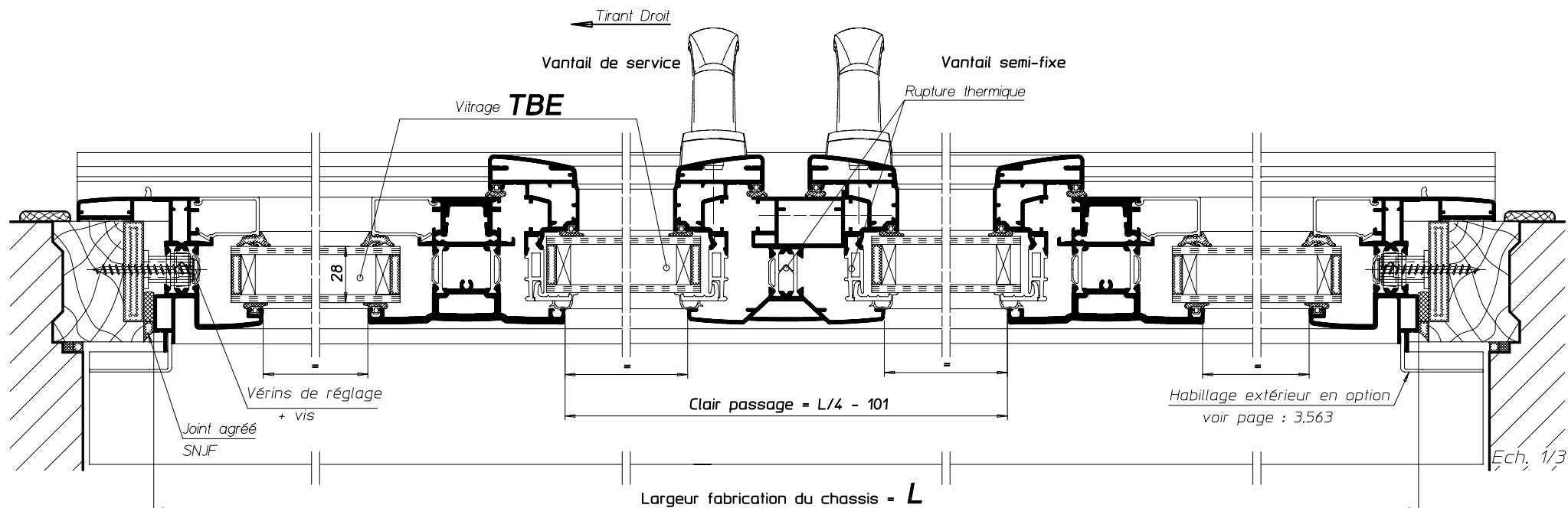
COUPE HORIZONTALE
