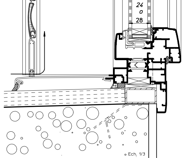
SECCIÓN VERTICAL
