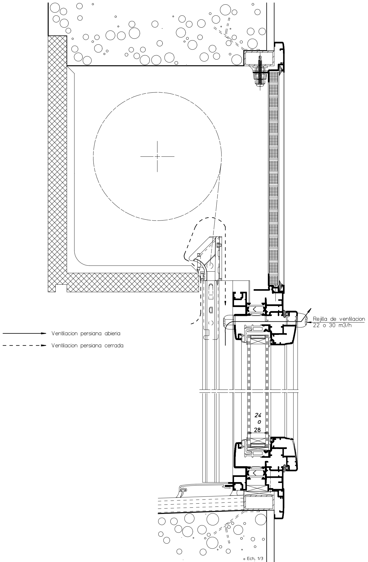
SECCIÓN VERTICAL
